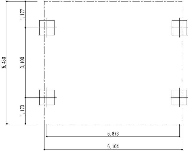
■ 基礎配置図
